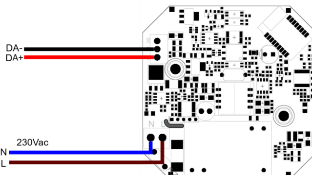
CABLAGGIO VERSIONE DALI
